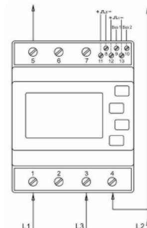
3 fas med N leder
