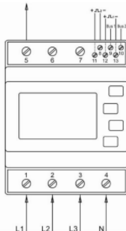
3 fas uten N leder
